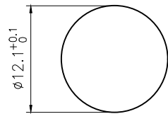
面板开孔尺寸
